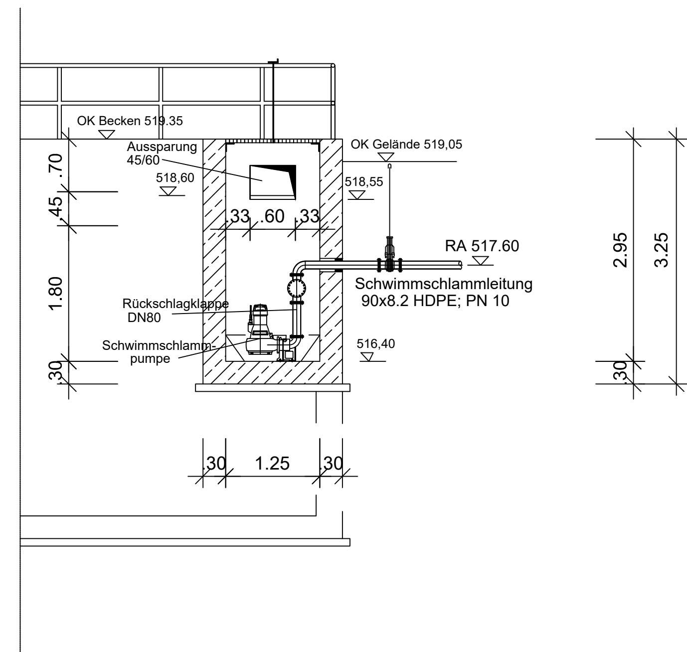
Schnitt D-D (Schwimmschlammumpenschacht)
