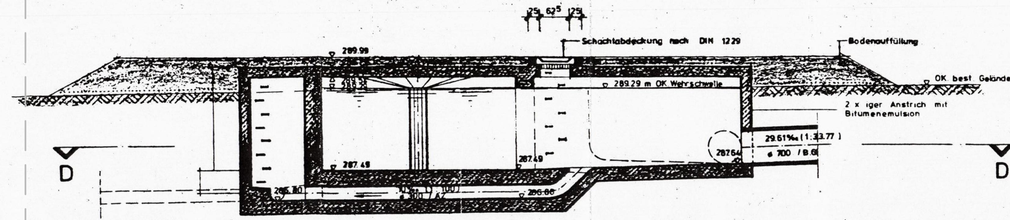
Schnitt A-A
