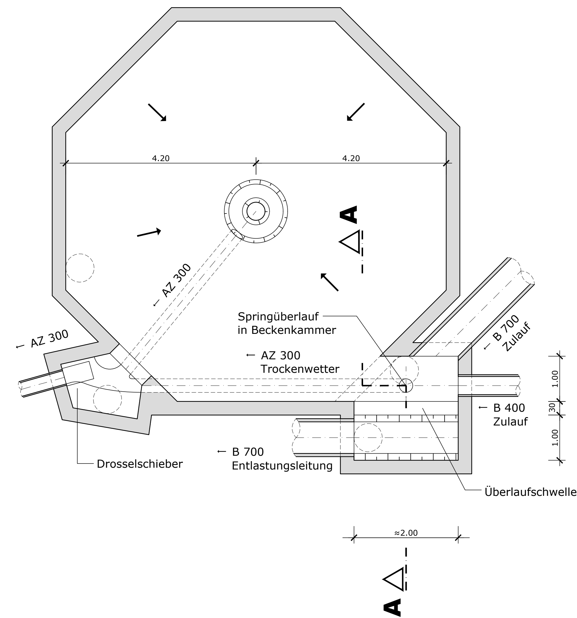
Grundriss (Bestandsaufmaß)
