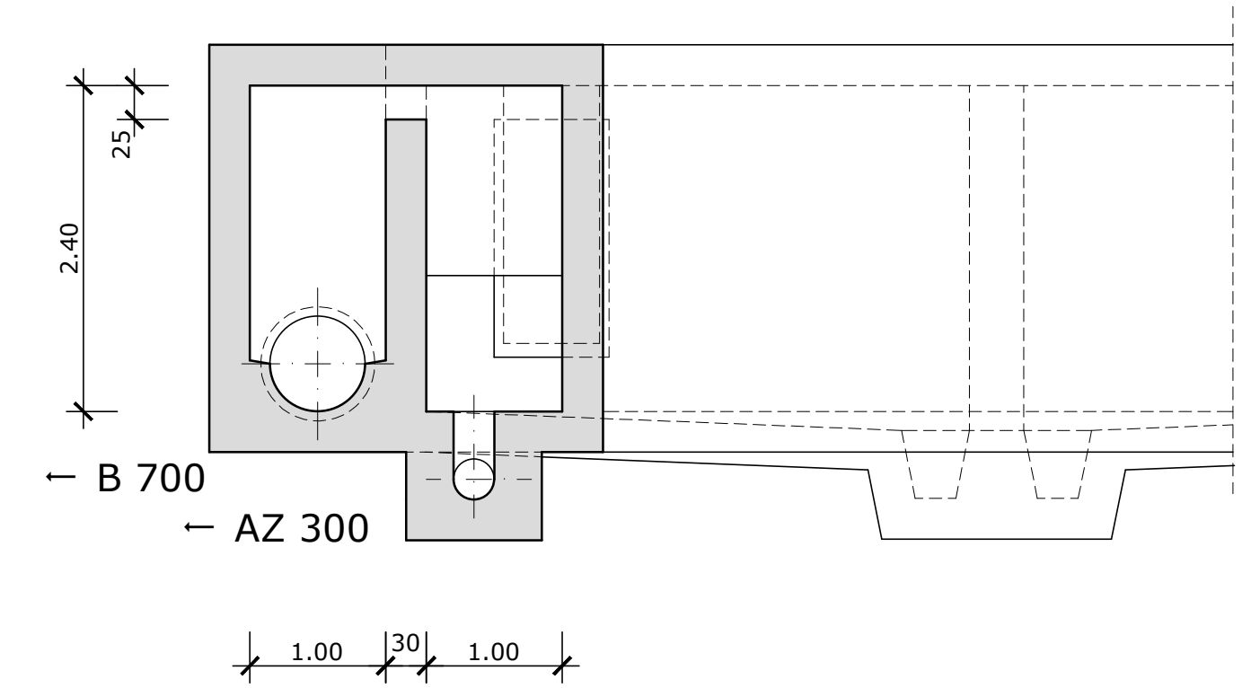
Schnitt A-A (Bestandsaufmaß)
