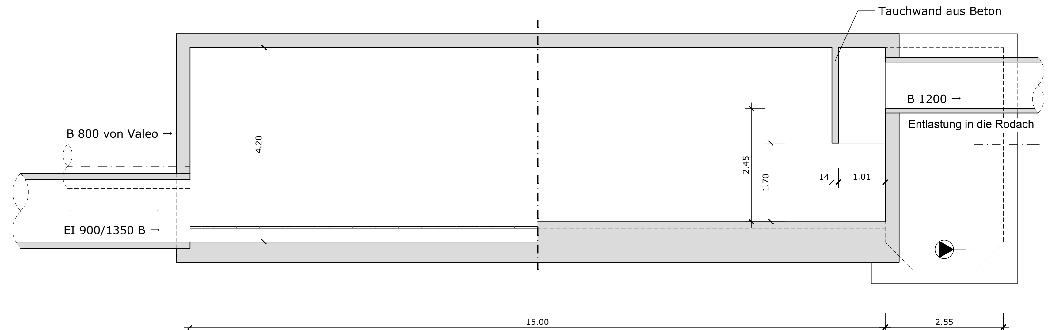
Schnitt A-A (Bestandsaufmaß)
