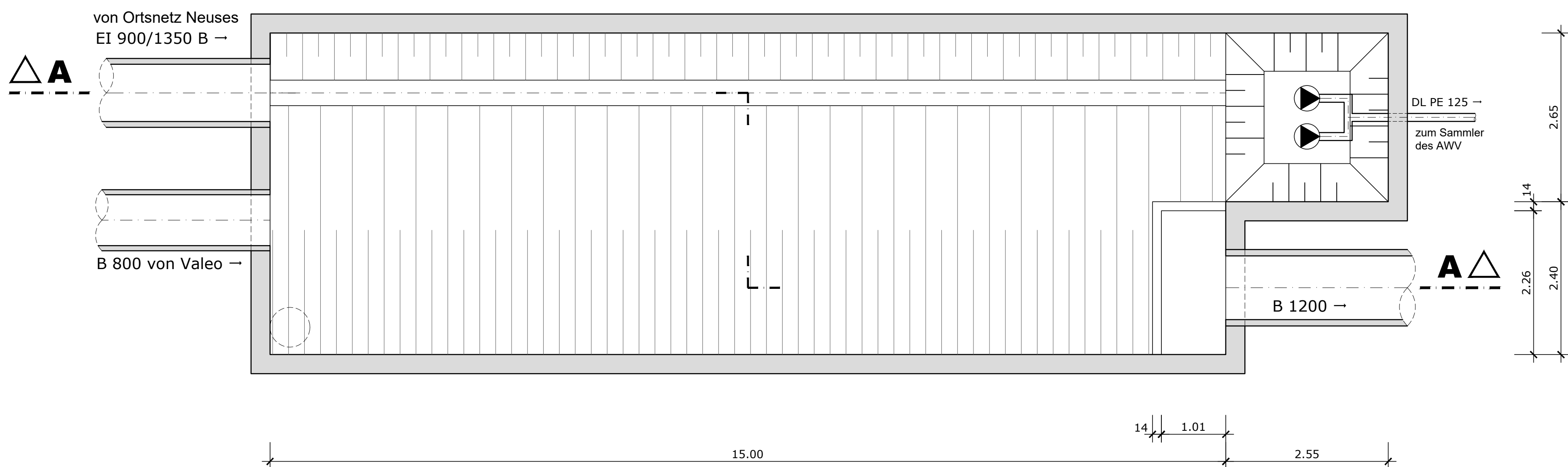
Grundriss (Bestandsaufmaß)
